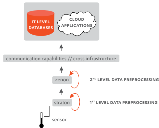
Abbildung 2: „On-the-fly“-Datenverarbeitung auf verschiedenen Ebenen mit zenon und straton.
