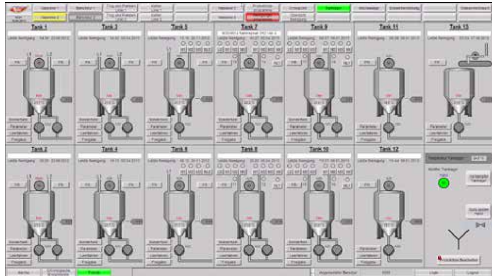
Die auf zenon basierende Anwendung verschafft den iglo-Mitarbeitern im Werk Reken einen Überblick über die Tanks und deren Füllstände.
