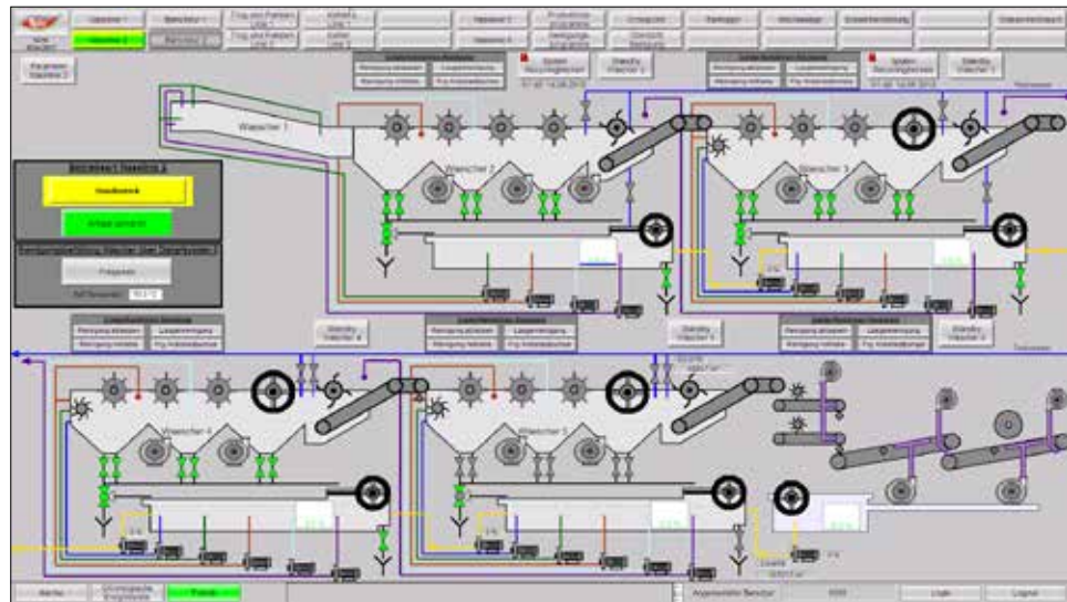
In drei Schritten wird das Gemüse gekühlt. Soll- und Ist-Temperaturen sind hierbei die wichtigsten Parameter für die Überwachung und Steuerung der Anlage.
