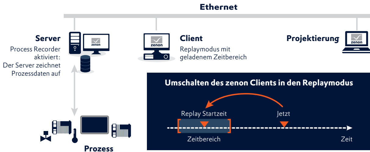
Abbildung 1: Funktionsweise des zenon Process Recorders.
