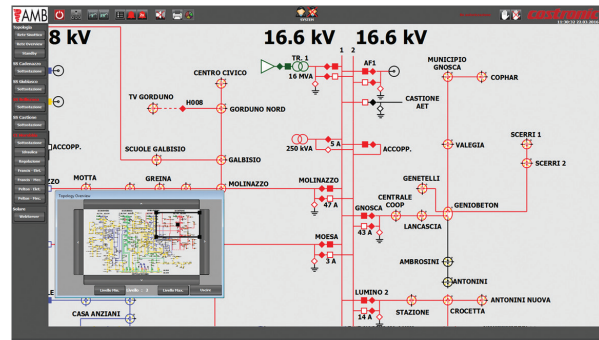
Abbildung 4: In einem zenon Weltbild werden alle Leitungen und Stationen angezeigt. Dabei kann der Ausschnitt beliebig gezoomt und verschoben werden.
