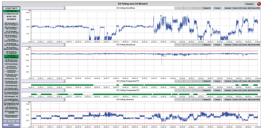
Abbildung 3: Die mit der Faceplate-Technik in zenon geschaffene Trend-Lösung erhöht die Benutzerfreundlichkeit.
