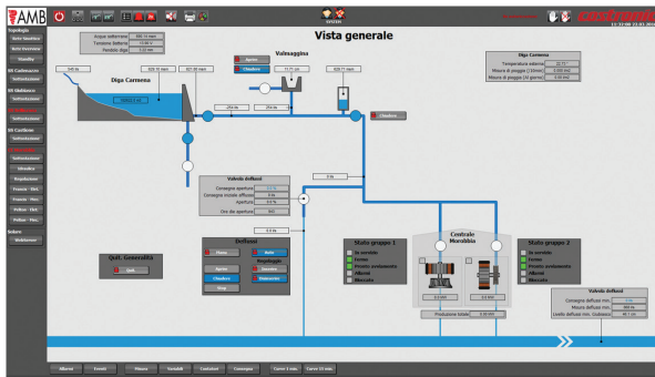
Abbildung 3: Abläufe und Zustände der Turbinen lassen sich mit einem Blick erfassen. Bei Bedarf können die Mitarbeiter problemlos Details anzeigen lassen.
