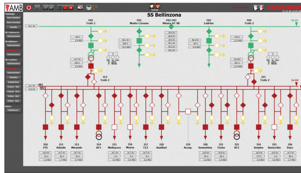
Abbildung 2: Bei der Verteilung von 50 kV auf 16 kV wird der Zustand jeder Leitung über ALC exakt angezeigt.
