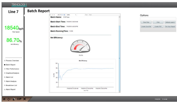
Abbildung 3: Berichte können in sehr kurzer Zeit erstellt werden. Praktisch alle Details können auf Chargenebene angezeigt werden.
