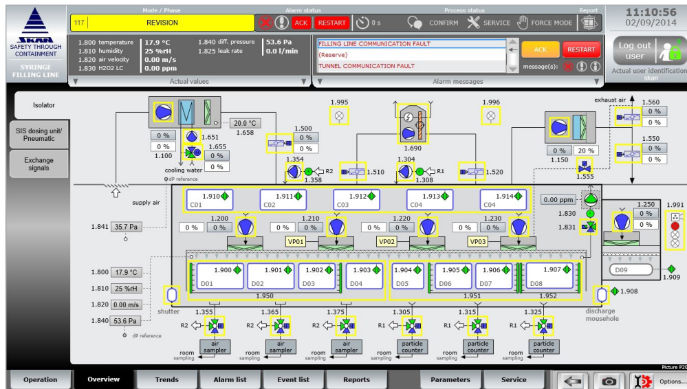
Abbildung 2: Perfekter Überblick: Die vielen Anlagenkomponenten sind mit einem Blick überschaubar und das erleichtert die schnelle Fehlerortung.
