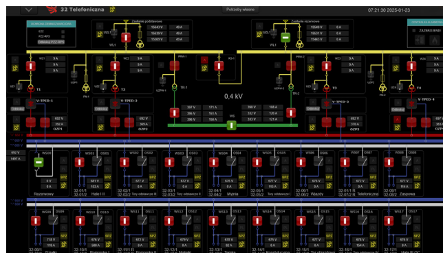
Schemat wizualizacji stacji elektroenergetycznej z podziałem na transformatory, pola rozdzielcze i linie zasilające. Operator ma możliwość monitorowania przepływów prądu i napięć w poszczególnych sekcjach oraz kontroli stanu zabezpieczeń i wyłączników.
